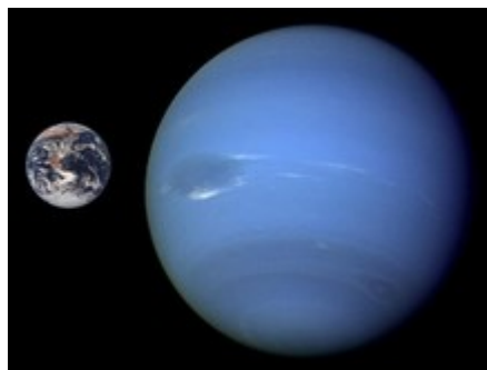
Comparaison entre Neptune et la Terre Photo : wikipedia.org
